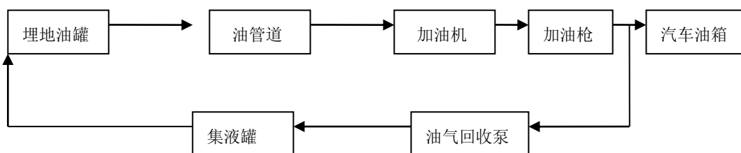
图 2-3 汽油加油工艺流程示意图
