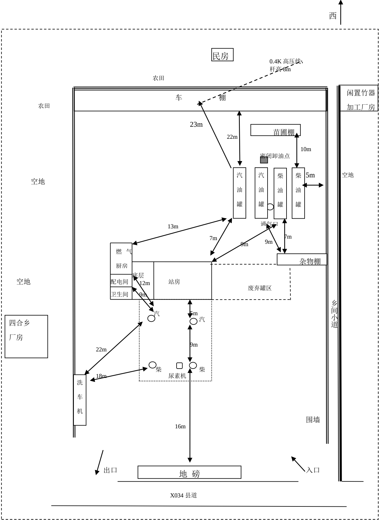
9.1 总平面布置示意图（2025.03）
