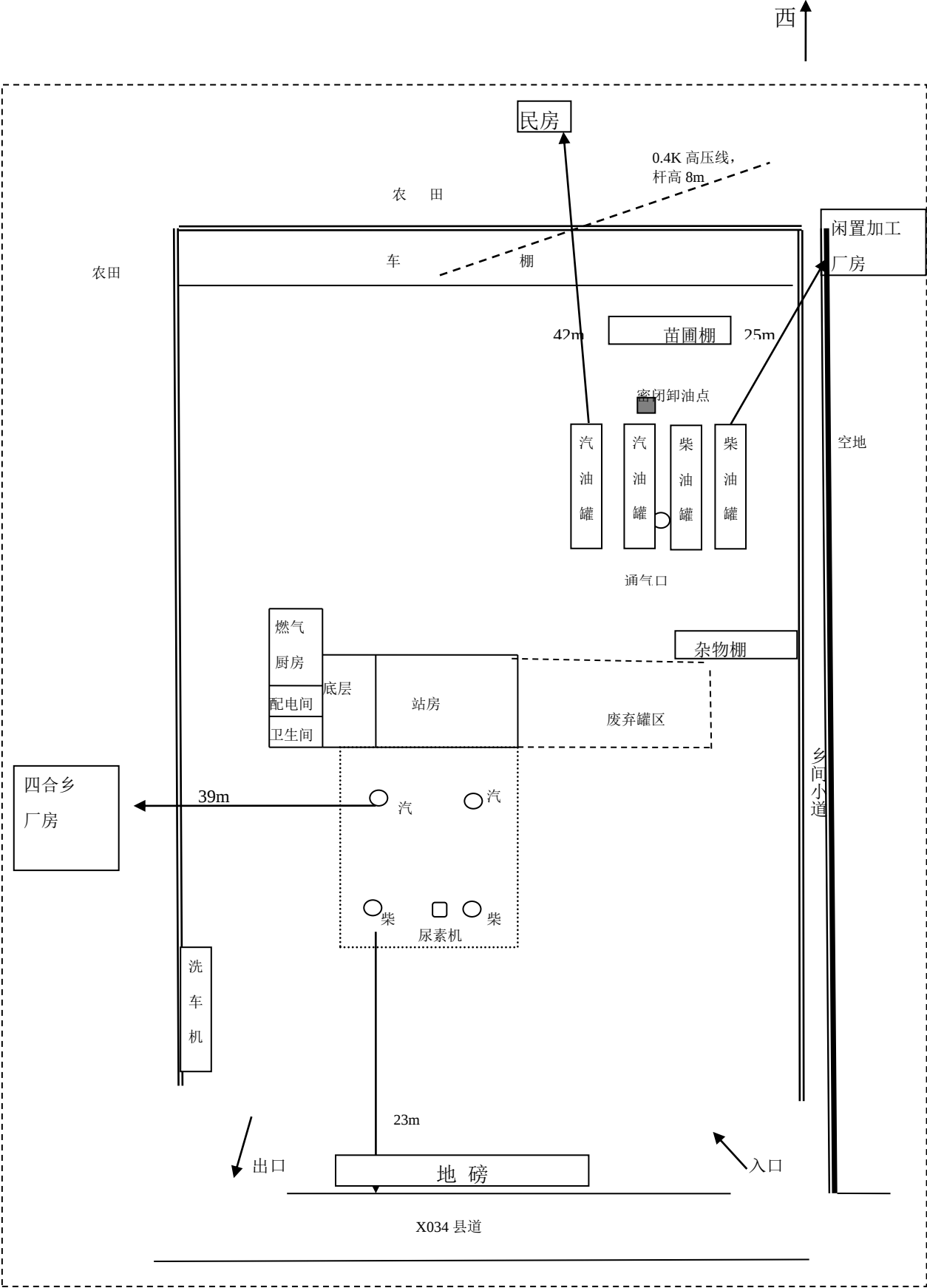
9.2 周边环境示意图（2025.03）
